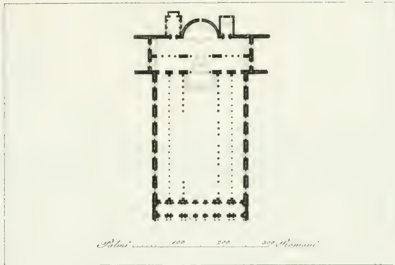
Pianta della Basilica di S. Pietro.
